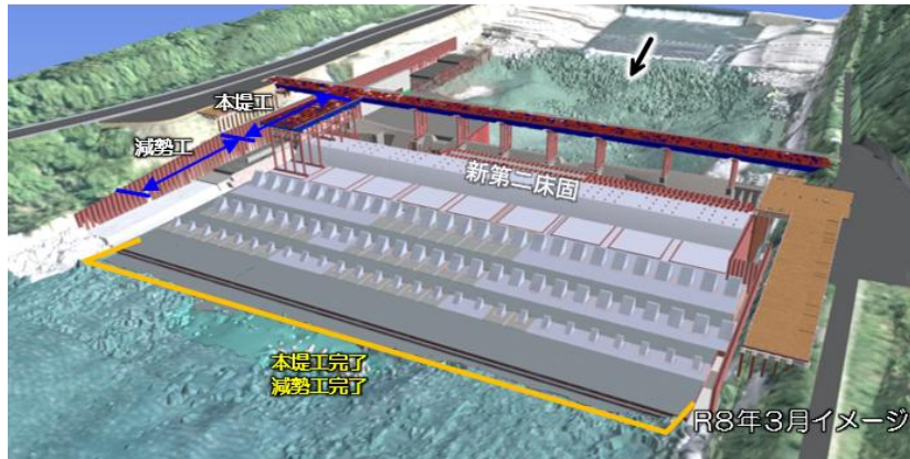
図4 第二床固改築工事の進捗状況
