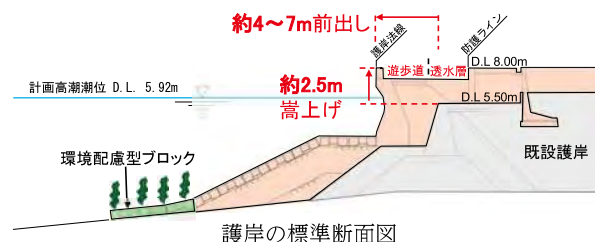
護岸の標準断面図
