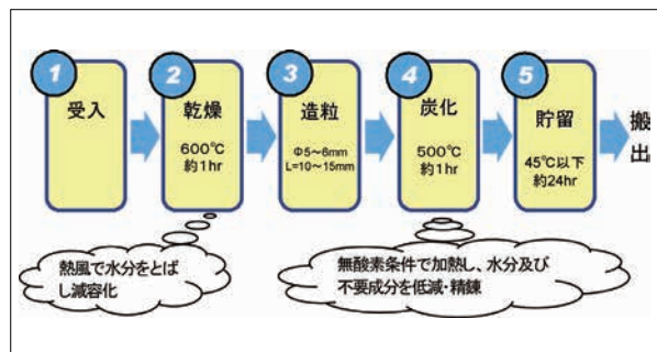
下水汚泥燃料化の処理フロー 脱水ケーキ100t/日から約8t/日の燃料を製造可能
