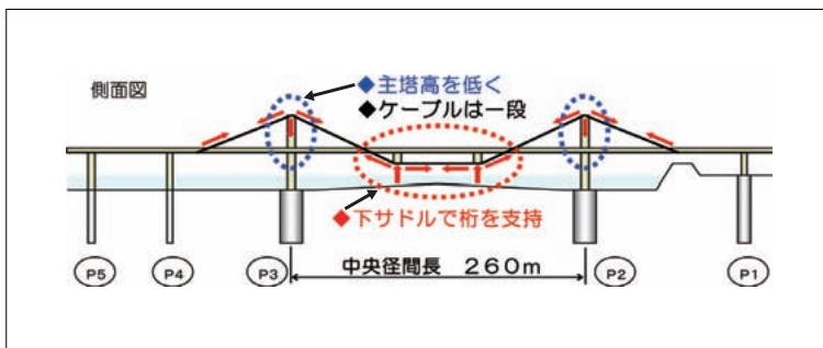
干潟部の上部工にケーブルイグレット形式を採用
