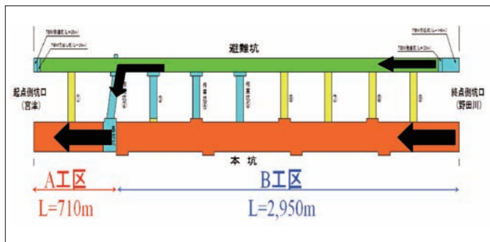
避難坑を活用した同方向2切羽による工期短縮
