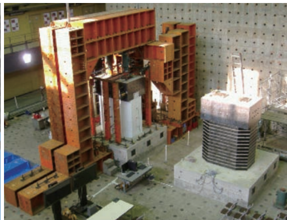
鶴見つばさ橋中空SRC橋脚の炭素繊維シート補強効果確認模型試験
