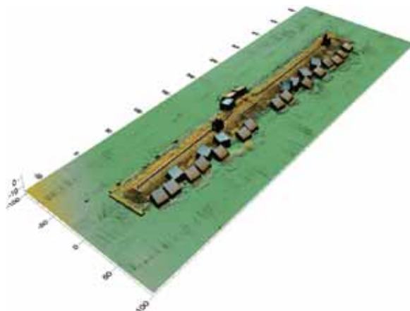
マルチビームソナーによる被災状況図
