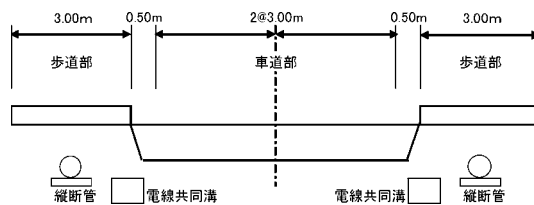
標準断面図
