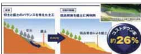
低品質岩を道路盛土へ再利用
