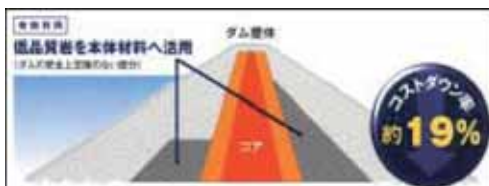
低品質岩をダム堤体盛土に活用
