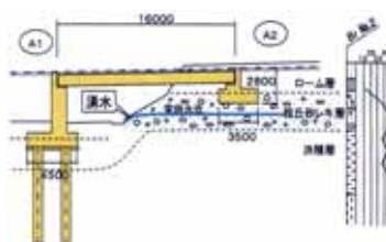
橋梁形式
