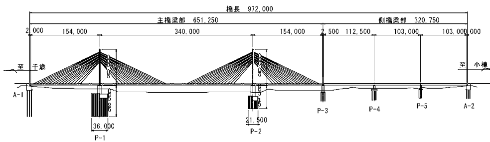
美原大橋橋梁一般図
