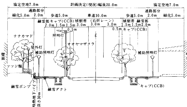
標準横断面
