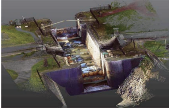
3Dレーザ測量（橋梁、ゲート非表示） 施設の現状、設計及び施工監理を把握し、文化財補修の記録に寄与できた
