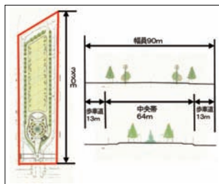
平面図・断面図
