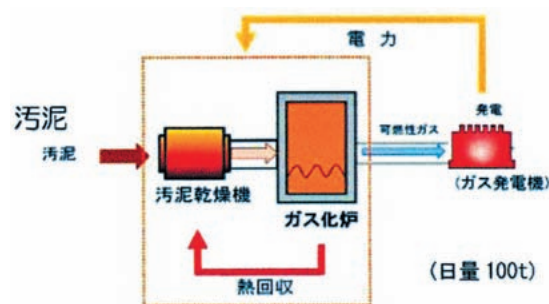
下水汚泥ガス化炉概略フロー
