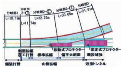
分岐部平面図
