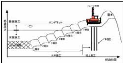
第2工区地盤改良概念図
