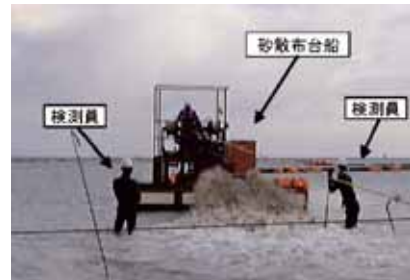
敷砂（水搬施工）状況
