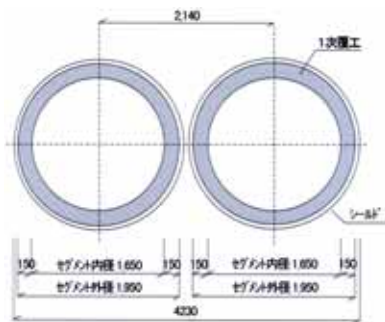
導水路標準断面図
