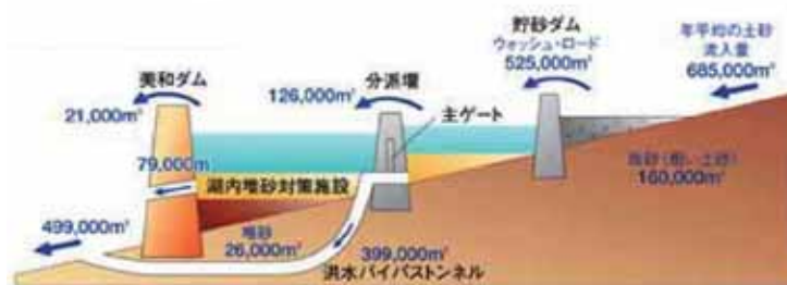
土砂移動量図（年間）
