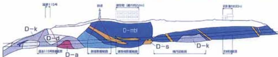
横道トンネル地質縦断面図
